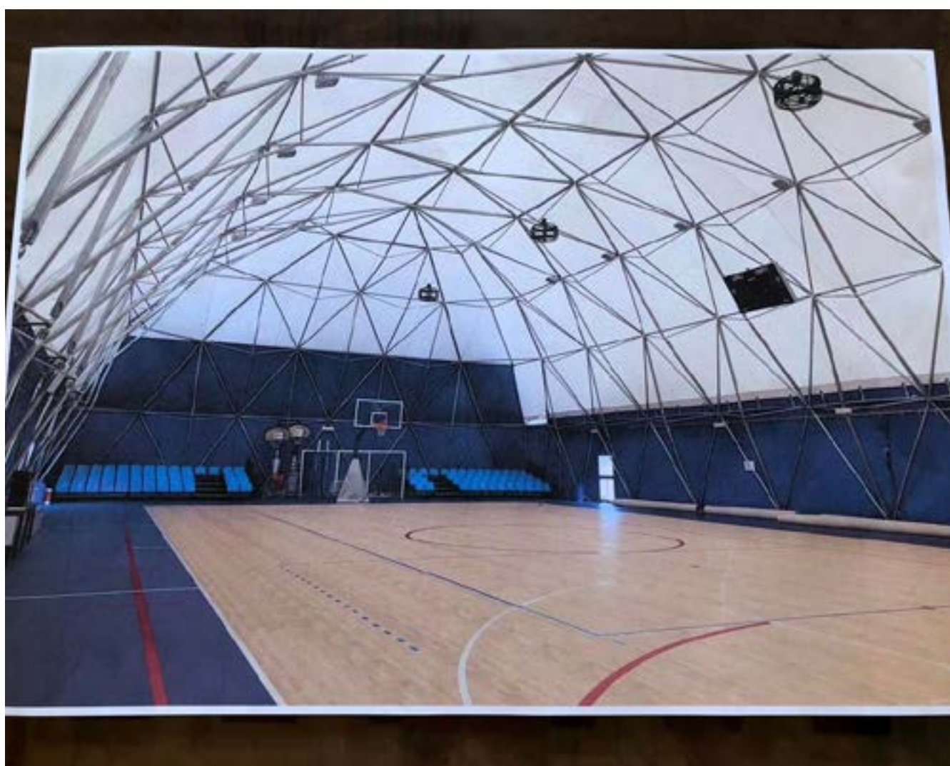
Ανάλογο κλειστό γήπεδο - θόλος - κατασκευάστηκε στην Καρδάμaina της Κω
